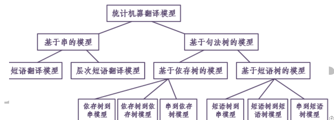
图 9 统计机器翻译典型模型
